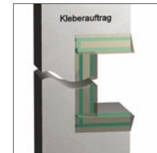
Obr. 2: Housenky lepidla na rozích
